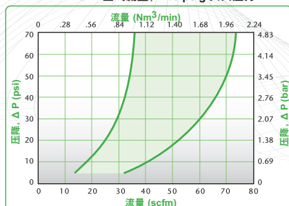
EFC12 空气流量, 100 psig 入口压力
