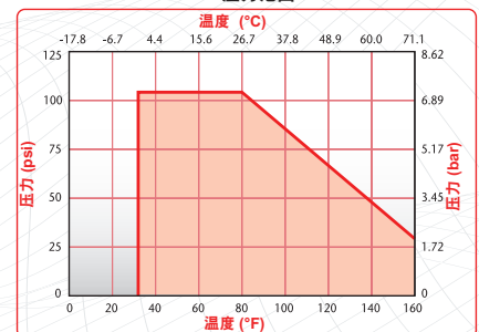
EF12 压力范围
