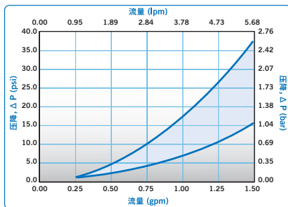
BLQ2 流量
